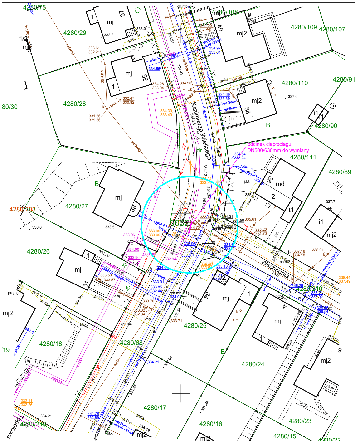
PLAN SYTUACYJNY SKALA 1:500 (sekcja mapy 6.120.30.18.2.4)
