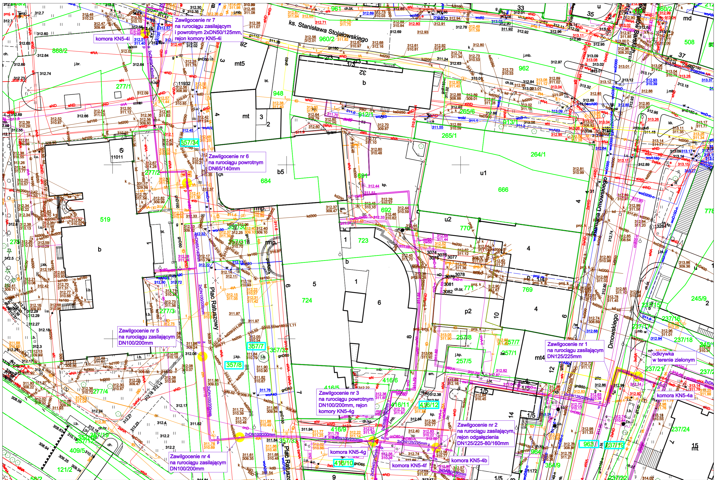
MAPA POGLĄDOWA - LOKALIZACJA ZAWILGOCENŃ NA SIECI CIEPŁOWNICZEJ W REJONIE UL. R.DMOWSKIEGO I PLACU RATUSZOWEGO W BIELSKU-BIAŁEJ SKALA 1:500
